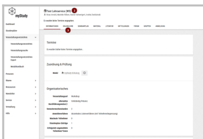
Fig. 3: Veranstaltungsansicht
