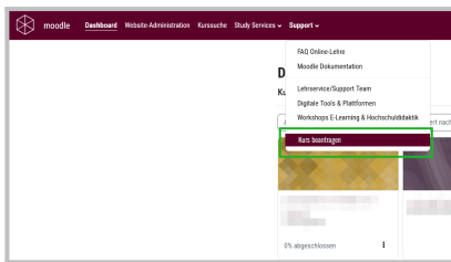
Fig. 6: Hauptnavigation
