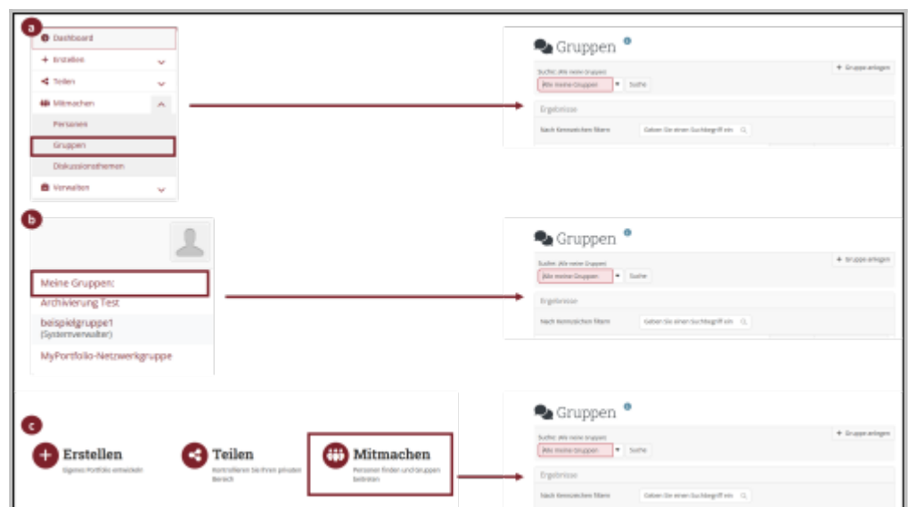
Abb. 1: Gruppen erstellen
