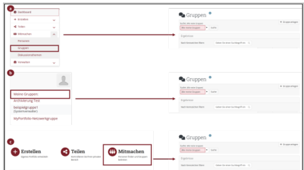
Abb. 2: Gruppen erstellen
