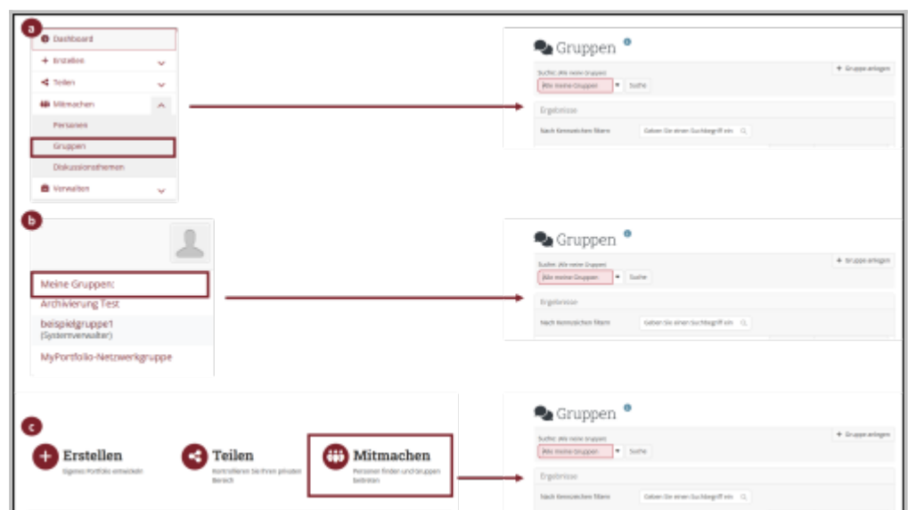
Abb. 1: Gruppen erstellen
