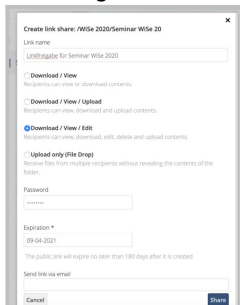
Abb. 5: Download-Rechte
