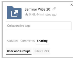
Abb. 4: Linkfreigabe
